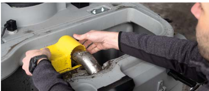
Filtre panier pour bloquer les éventuels déchets et éviter qu'ils ne se déposent sur le fond du réservoir de récupération.
